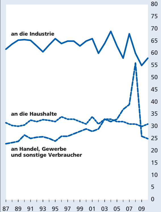
Entwicklung der Stromabgabe der öffentlichen Elektrizitätsversorgungsunternehmen 1987 – 2010
