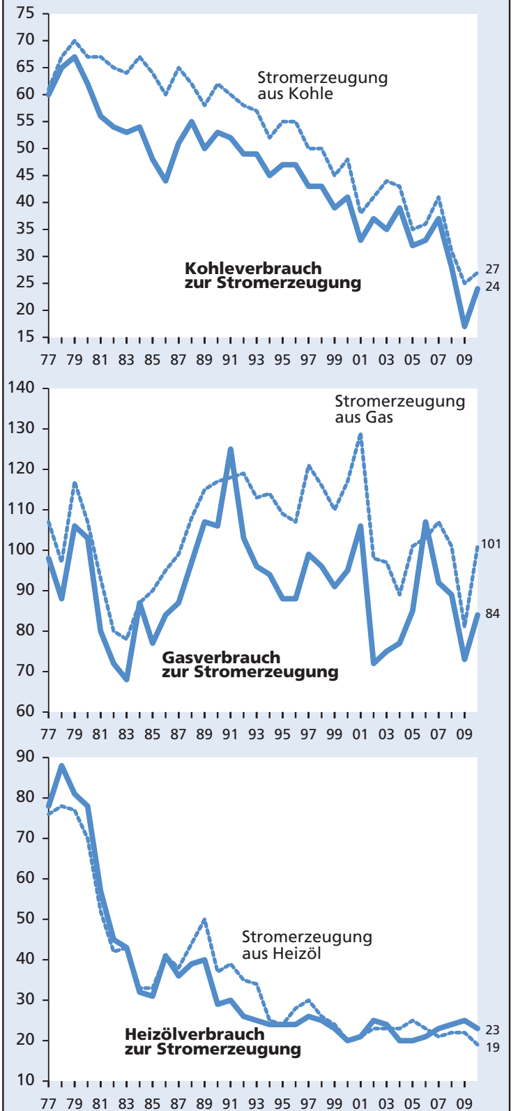
Entwicklung des Verbrauchs der Einsatzstoffe zur Stromerzeugung durch Stromerzeugungsanlagen des Verarbeitenden Gewerbes sowie des Bergbaus und der Gewinnung von Steinen und Erden 1977 – 2010
