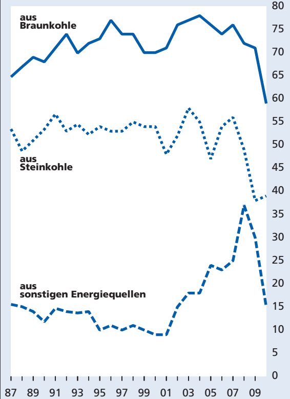
Entwicklung der Stromerzeugung der öffentlichen Elektrizitätsversorgungsunternehmen 1987 – 2010
